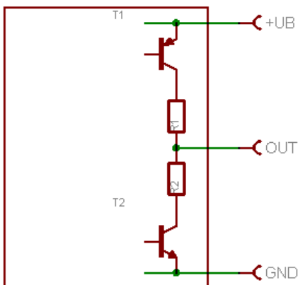
Abbildung 1 - Primäre Ausgangsstufe des SRZ
