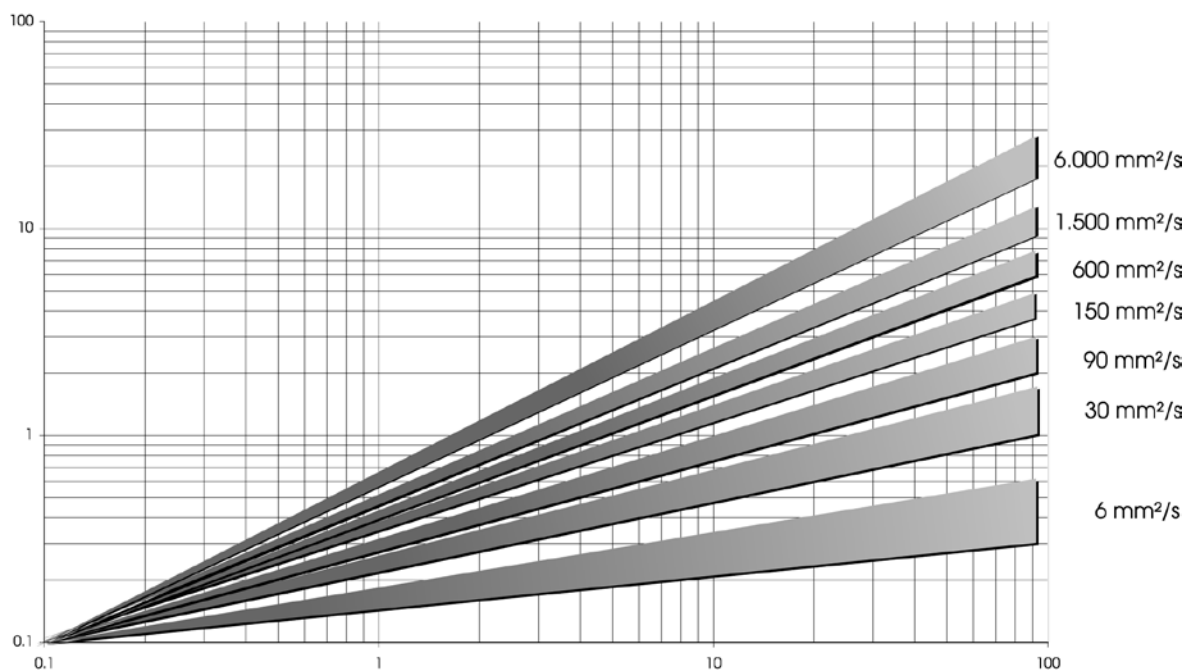
Abbildung 2 - Druckabfall als Funktion des Durchflusses
